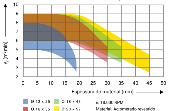
Valores indicativos para corte de aglomerado
